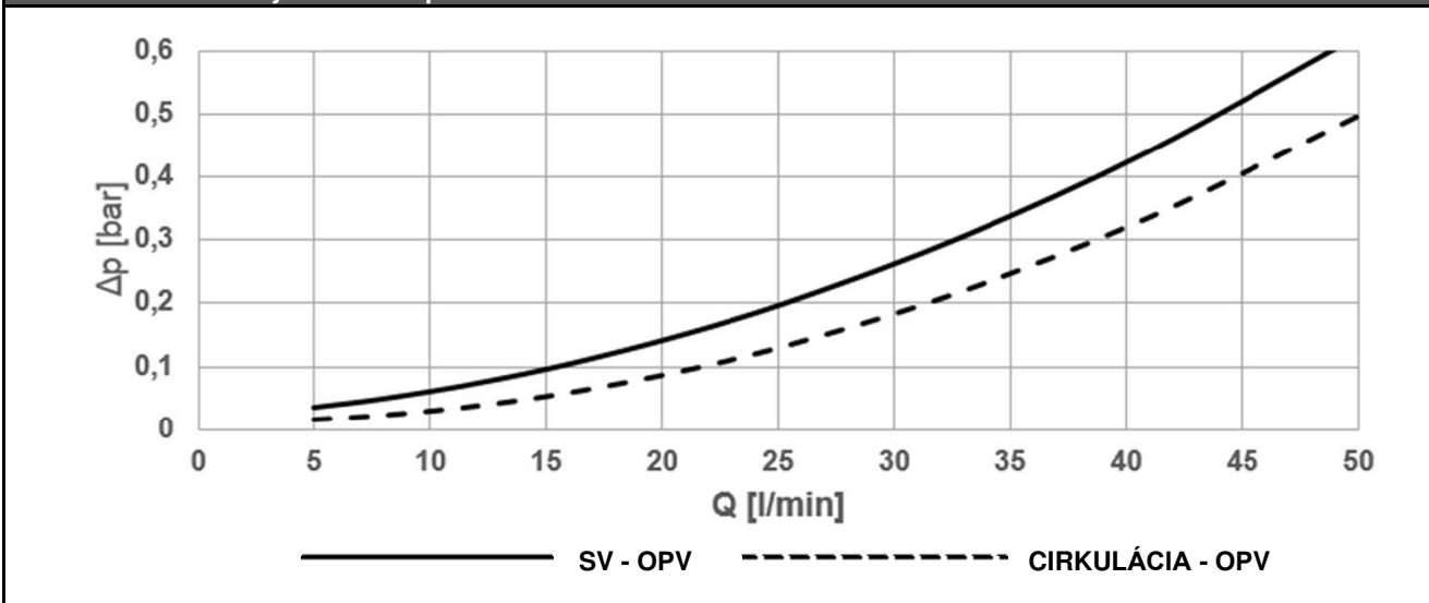
Graf závislosti tlakových strát na prítoku v zásobníku OPV
