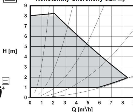
Konštantný diferenčný tlak \Delta p
