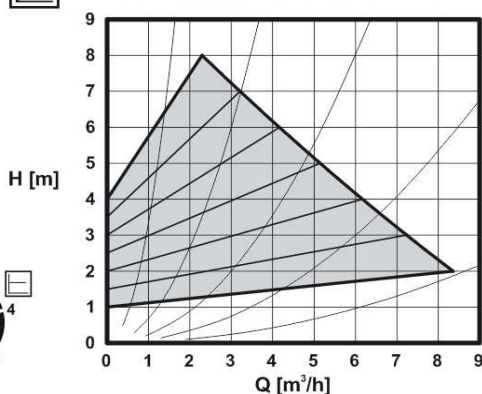
Premenný diferenčný tlak \Delta p
