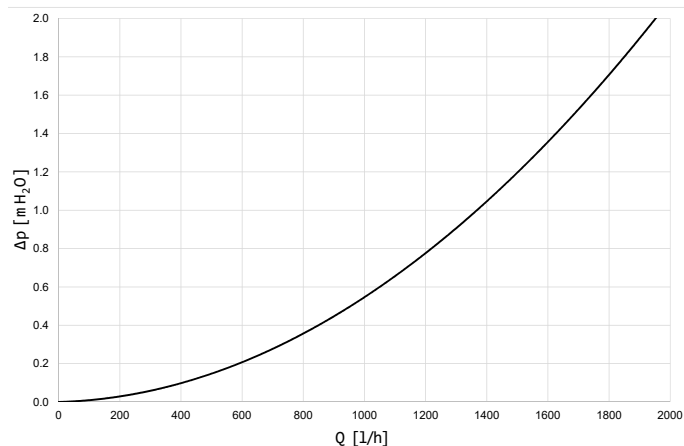
Graf tlakových strát jednotky RegulushBOX K – do vykurovacieho systému
