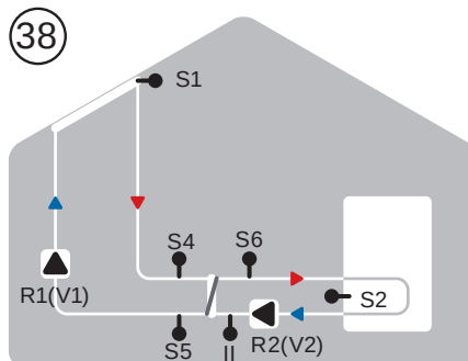
Solárny systém s výmenníkom +
