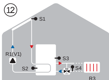
Solárny systém s vykurovacím okruhom
