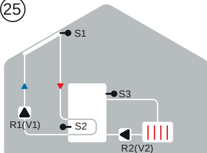
Solárny systém s chladením 3 (vychladenie kolektora)
