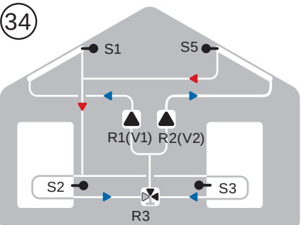
Solárny systém s 2 kolektorovými poľami (východ/západ), 2 zásobníky a 2 čerpadlami
