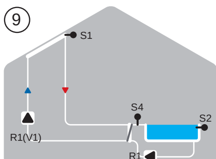
Solárny systém s bazénom a výmenníkom
