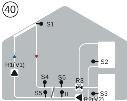
Solárny systém s výmenníkom a 2 zásobníkmi
