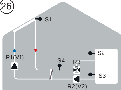
Solárny systém s výmenníkom, 2 zóny
