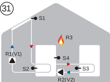
Solárny systém s odovzdávaním tepla medzi zásobníky a termostatom
