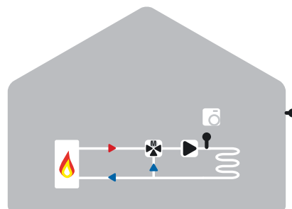
Zmiešavací vykurovací okruh s riadeným zdrojom
