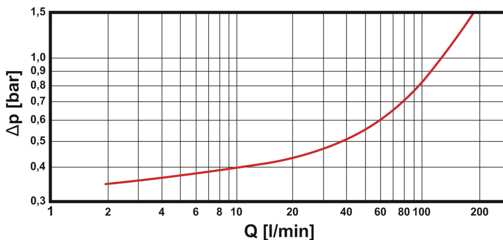
Graf tlakových strát
