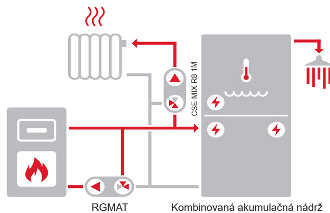
Príklad zapojenia II
