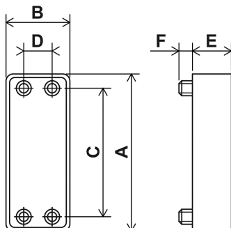
Rozmerová schéma
