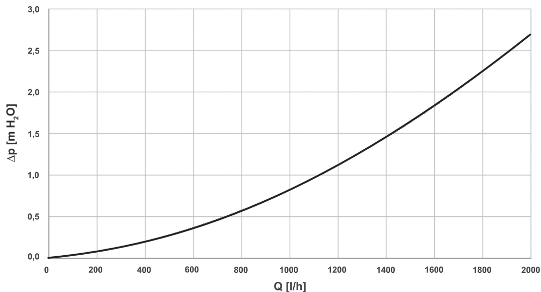
Graf tlakovej straty výmenníka
