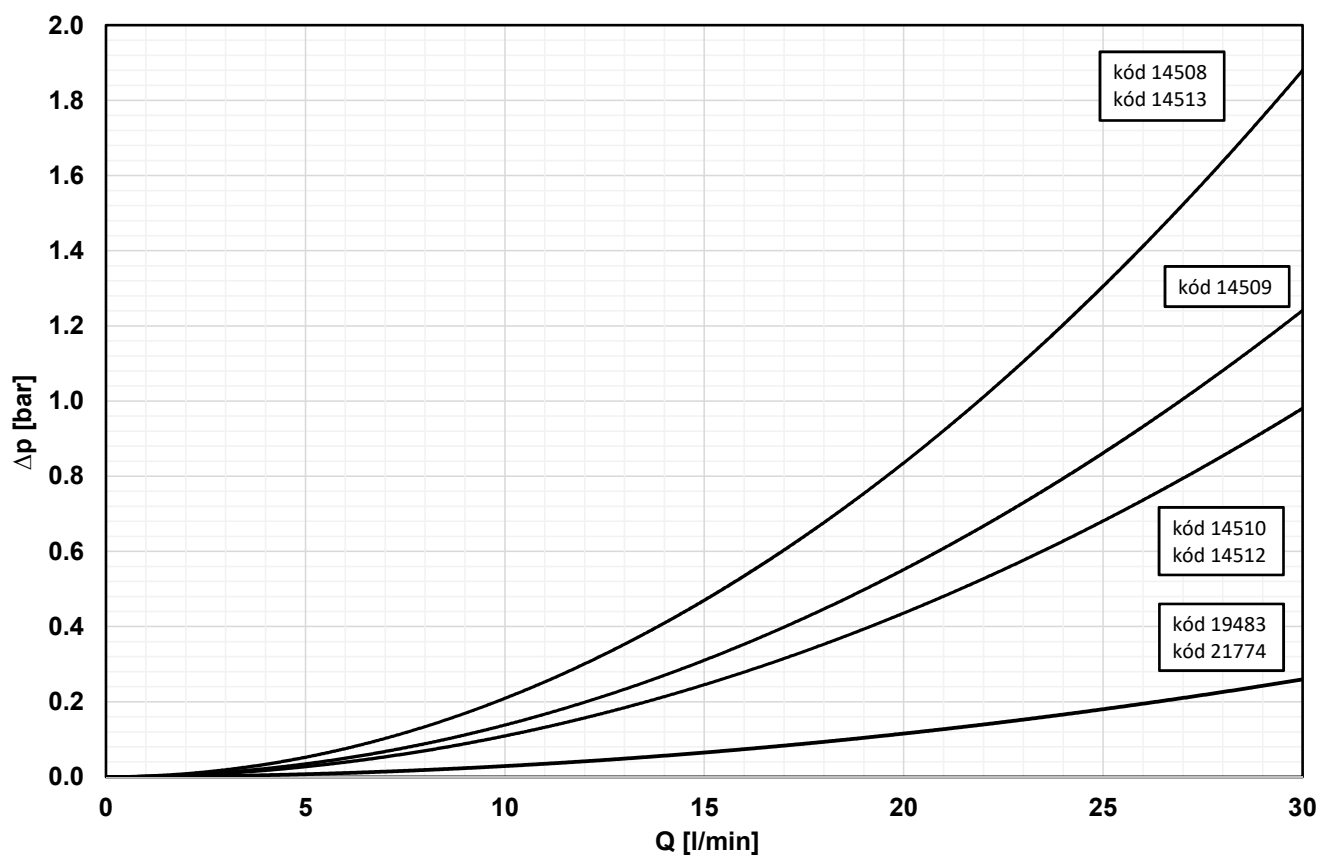
Graf tlakovej straty
