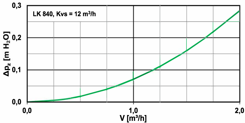
Graf tlakovej straty ventilu
