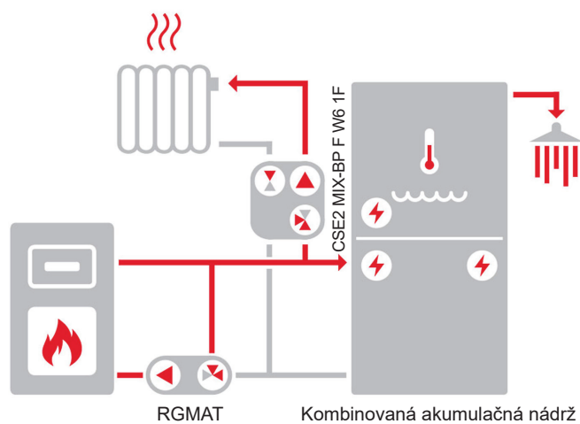
Príklad zapojenia
