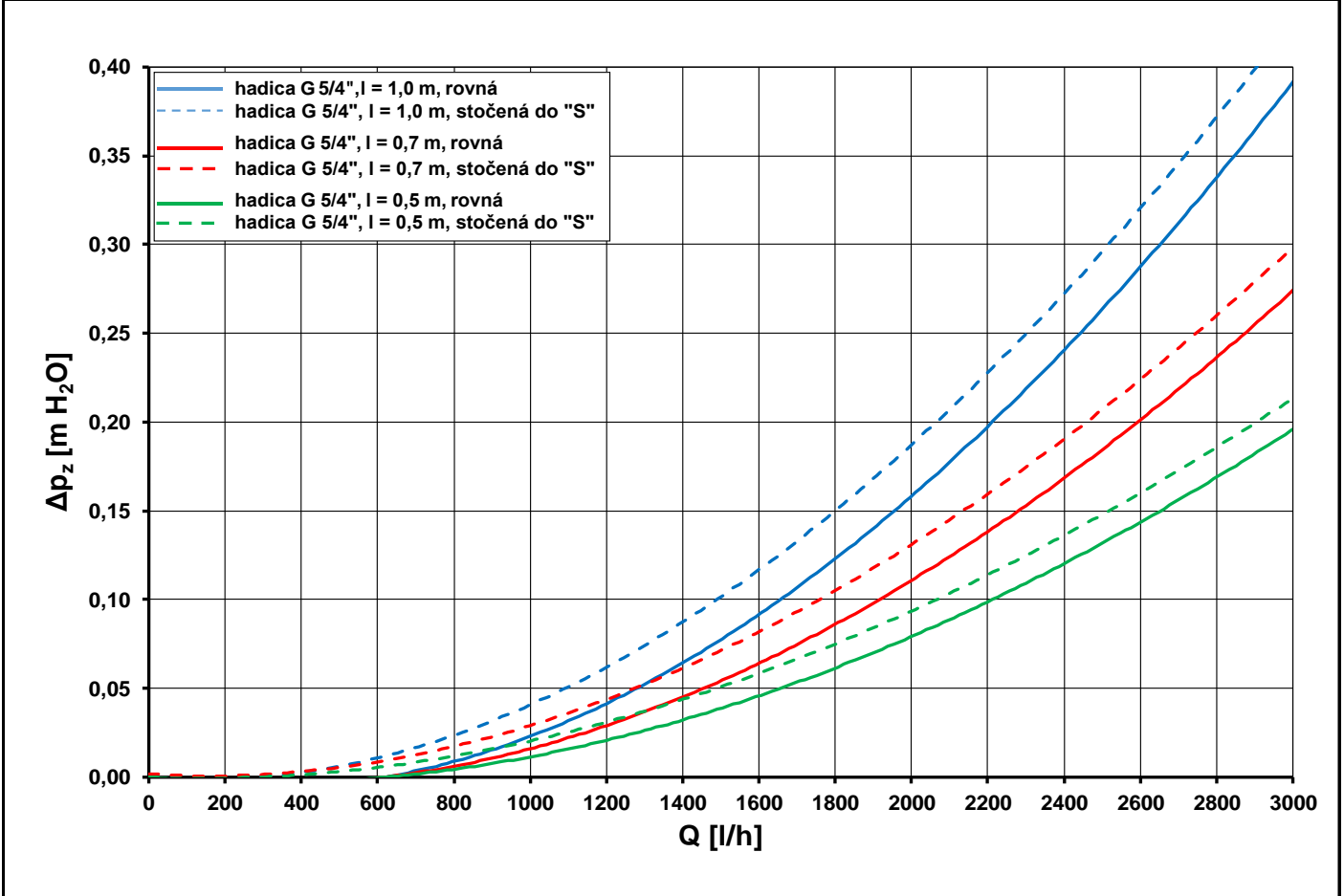
Graf tlakovej straty pre hadicu s pripojením G 5/4"
