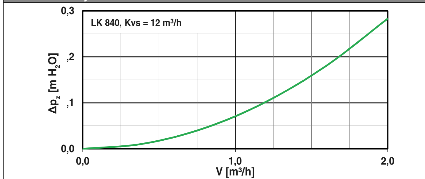
Graf tlakové ztráty ventilu
