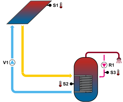
2. Solárny systém s cirkuláciou OPV
