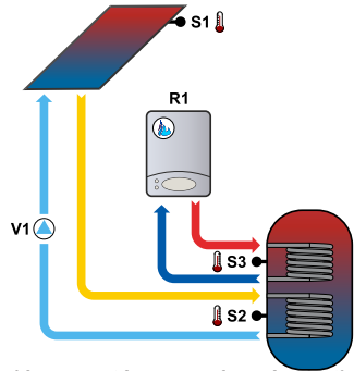
4. Solárny systém so spínaným kotlom
