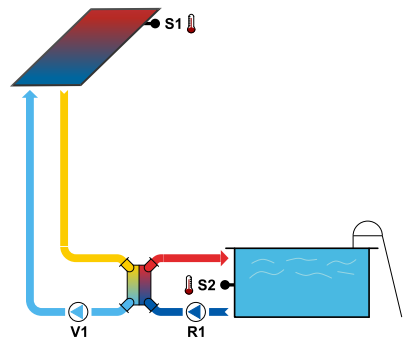
6. Solárny systém s výmenníkom a bazénom
