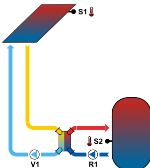
5. Solárny systém s výmenníkom
