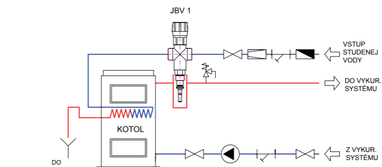
Obr. 4: Schéma inštalácie ventilu JBV1 do vykurovacieho systému s použitím spätnej klapky
