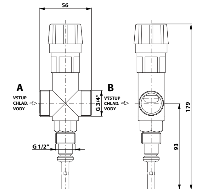
Obr. 1: Rozmerová schéma
