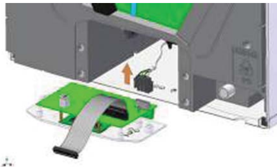
Obr. 7: Odpojenie 4pólového konektora (predná strana)
