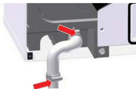
Obr. 11: Montáž hadice na kondenzát (zadná strana)
