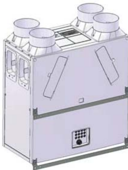
Obr. 19: Zadná stena s držiakmi na stene
