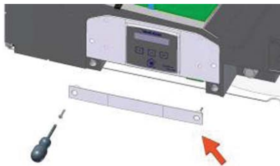
Obr. 4: Odmontovanie krytu elektrického panela (predná strana)
