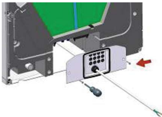
Obr. 8: Odmontovanie zadnej dosky s káblom (zadná strana)
