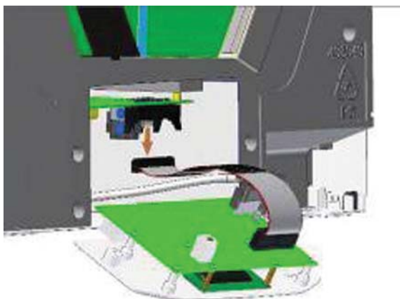
Obr. 6: Odpojenie plochého kábla (predná strana)
