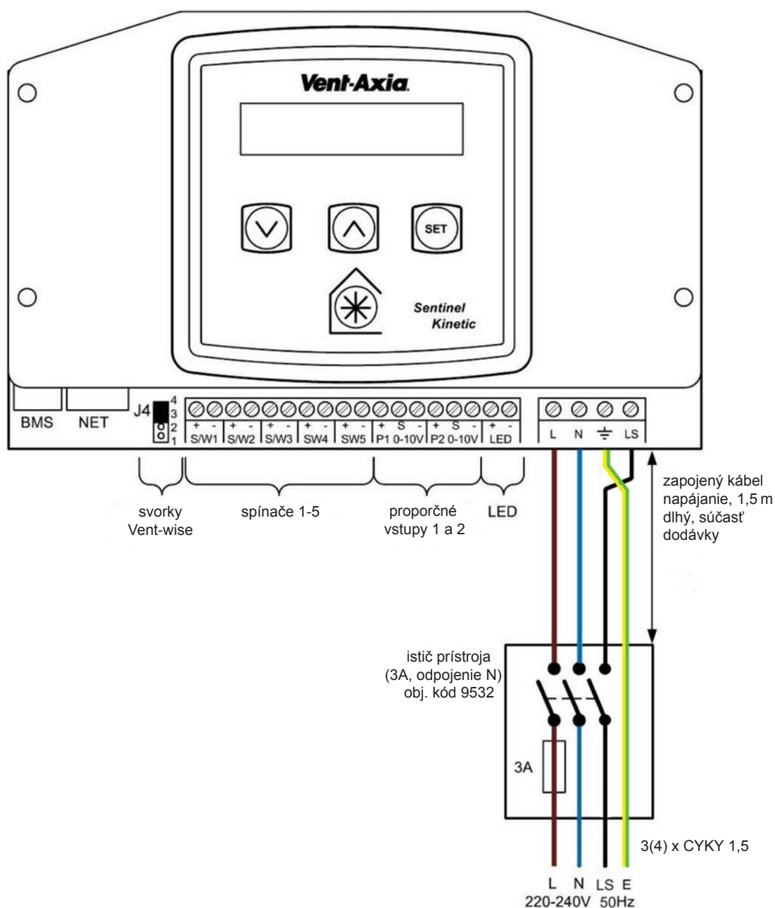
Obr. 23: Zapojenie svoriek
