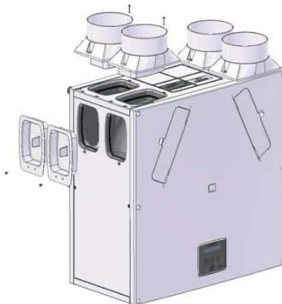
Obr. 18: Demontáž a inštalácia hrdiel
