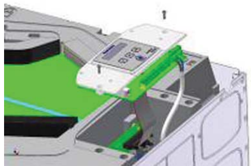
Obr. 5: Odpojenie kábla napájania (predná strana)
