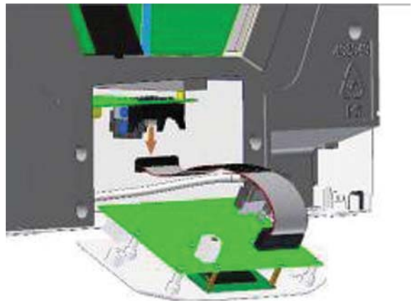
Obr. 6: Odpojenie plochého kábla (predná strana)
