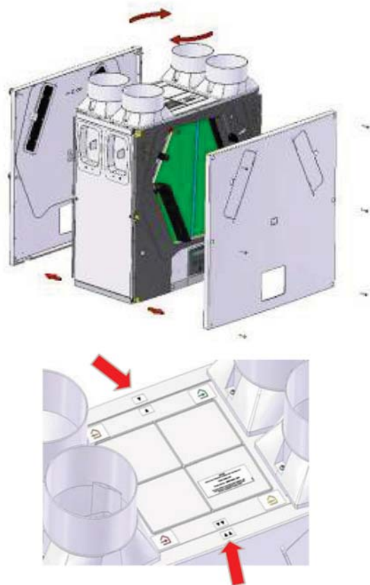
Obr. 3: Inštalácia prístroja v obrátenej polohe
