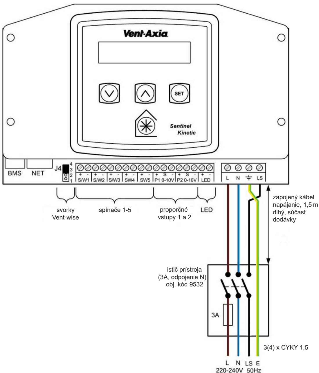
Obr. 23: Zapojenie svoriek
