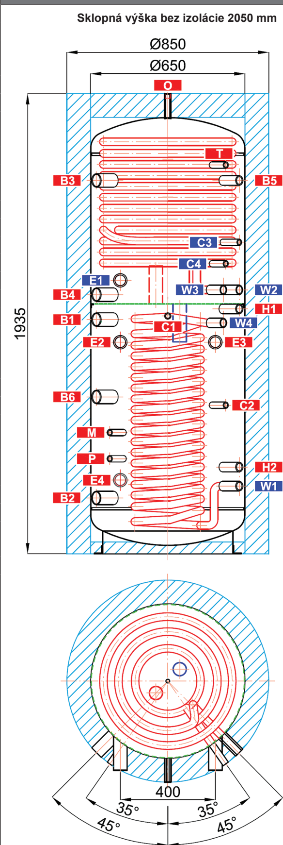
Rozmerová schéma
