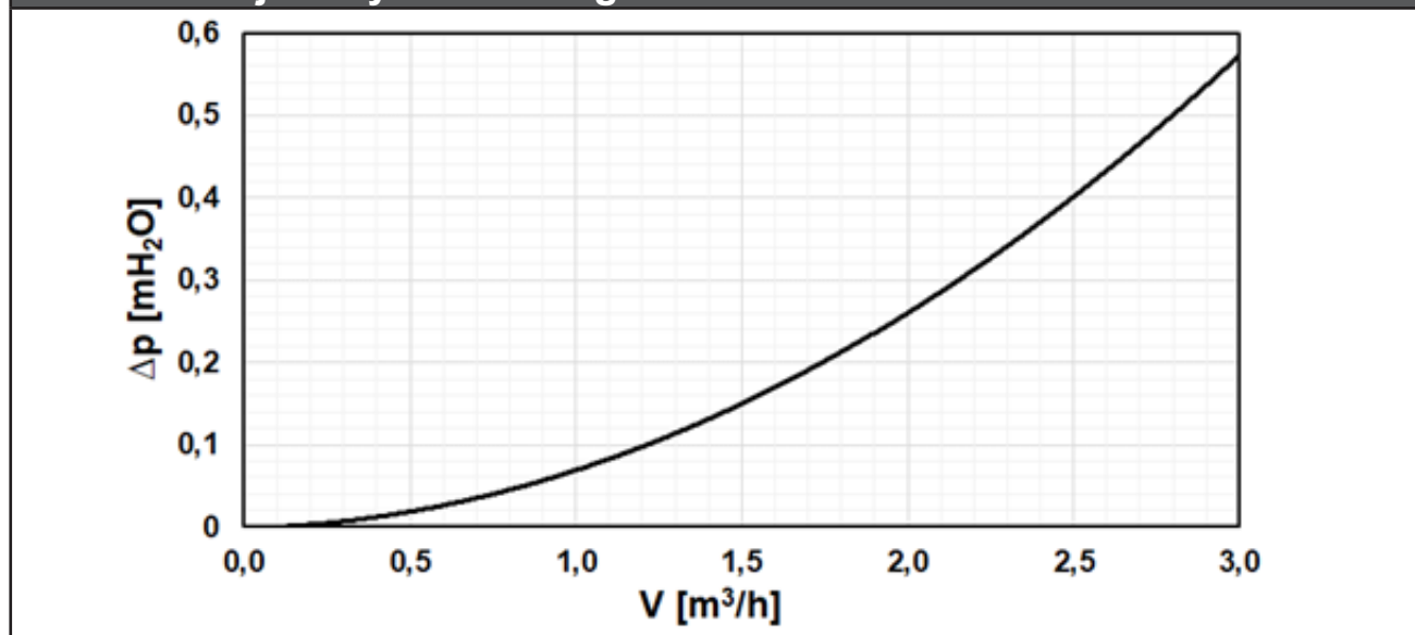
Graf tlakovej straty filtra s magnetom
