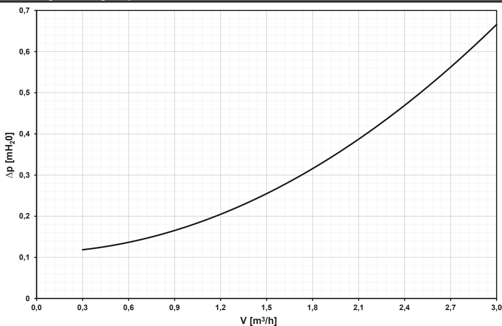
Graf tlakovej straty spätného ventilu
