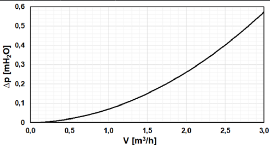
Graf tlakovej straty filtra s magnetom
