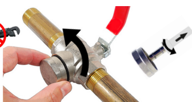
Obr. 7 - odskrutkovanie plastového krytu a vybratie filtračného sitka
