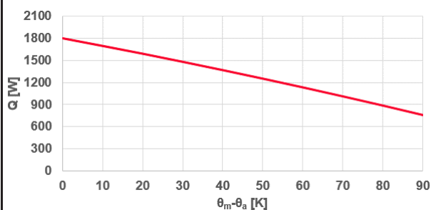
Graf výkonu kolektora
