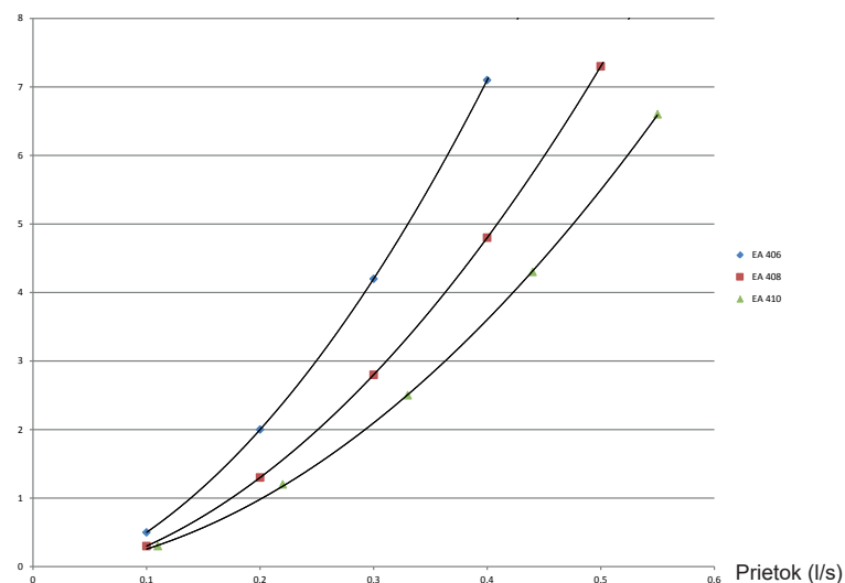
Graf tlakovej straty pre CTC EcoAir 400
