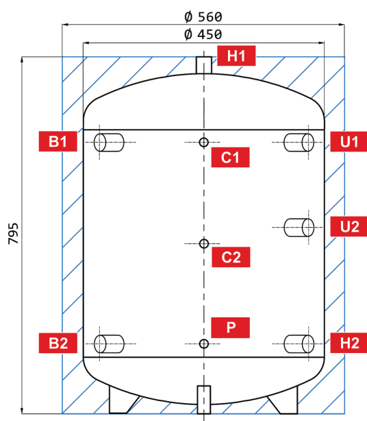
Rozmerová schéma
