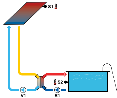
6. Solárny systém s výmeníkom a bazénom
