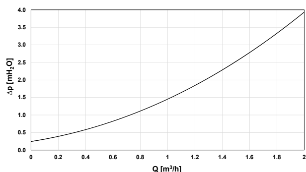
Graf tlakovej straty vykurovacieho systému
