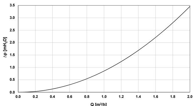
Graf tlakovej straty okruhu kotla
