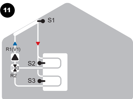
Solárny systém s vrstveným zásobníkom
