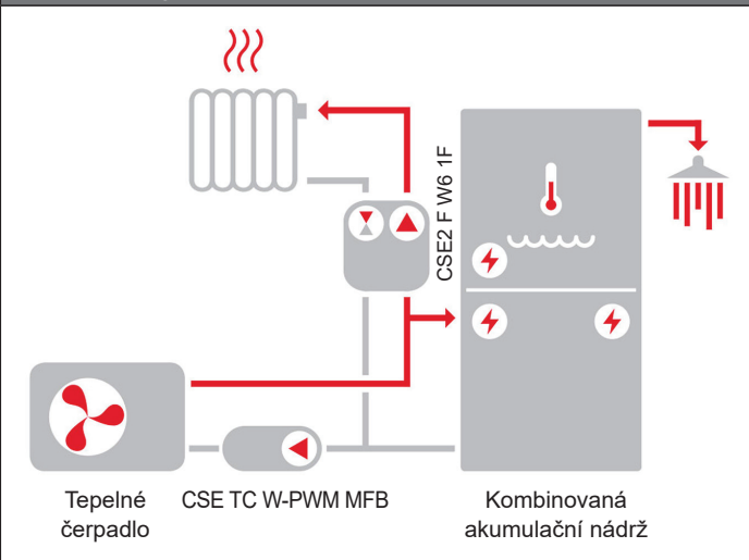
Příklad zapojení
