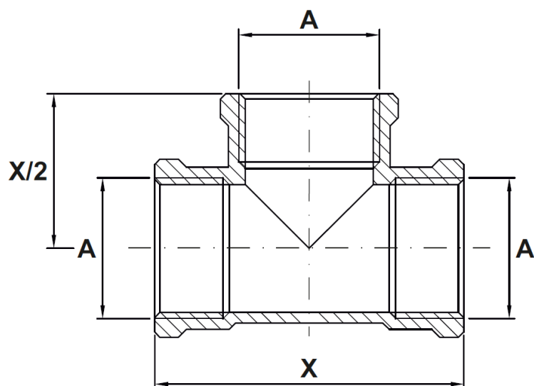
Rozmerové schéma
