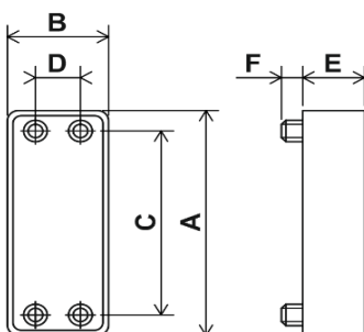
Rozmerová schéma
