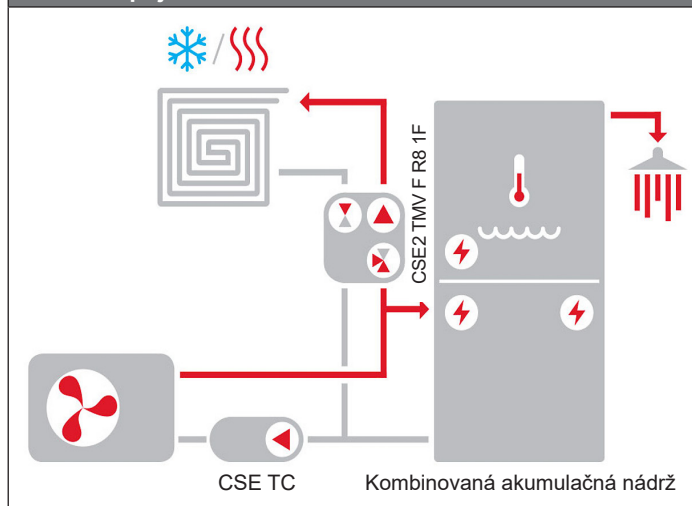
Príklad zapojenia II
