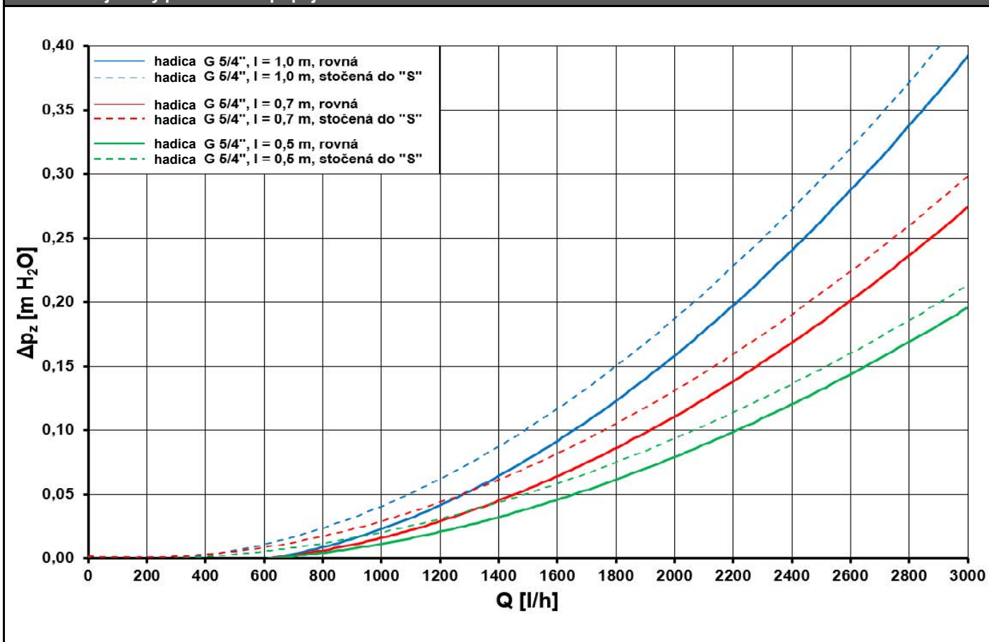
Graf tlakovej straty pre hadicu s pripojením G 5/4"
