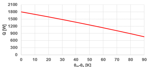
Graf výkonu kolektora
