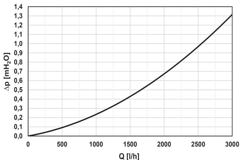
Graf tlakovej straty výmenníka
