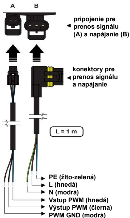
Pripojenie čerpadla UPM3 HYBRID
