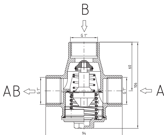
Rozmerová schéma
