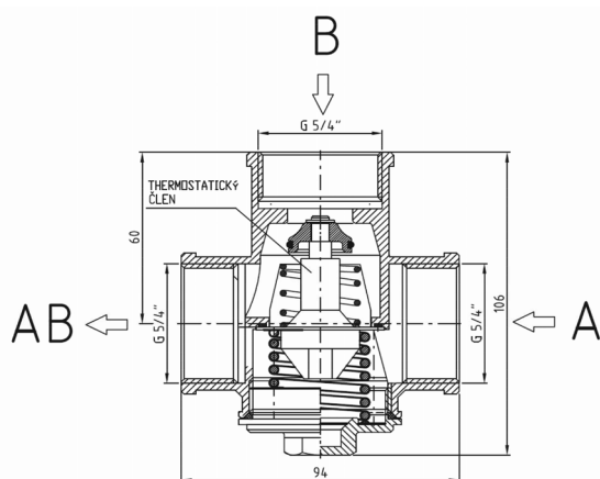
Rozmerová schéma
