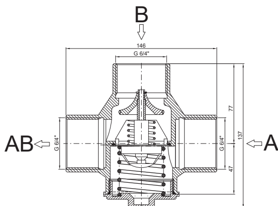
Rozmerová schéma
